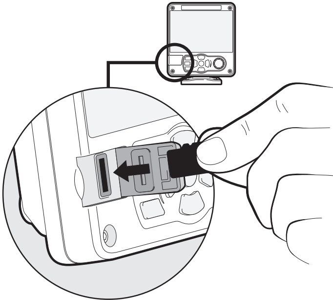
Figure 25 Port pour carte Micro SD
