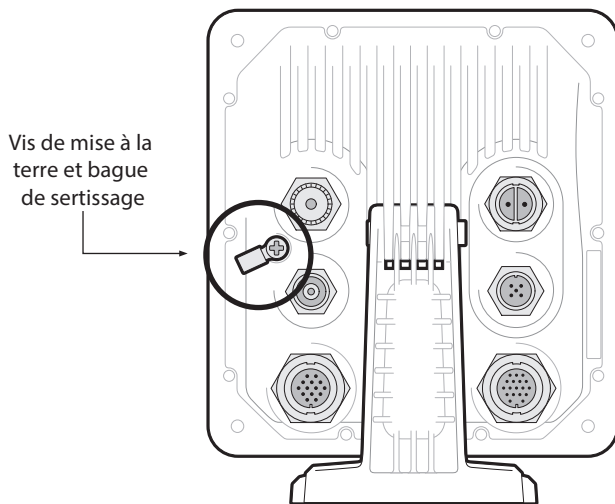
Figure 16 Mise à la terre de l'émetteur SIA
