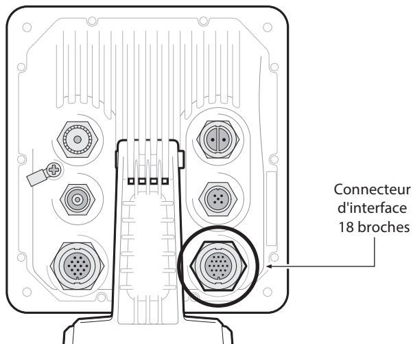
Figure 13 Connexion du port bidirectionnel de série
