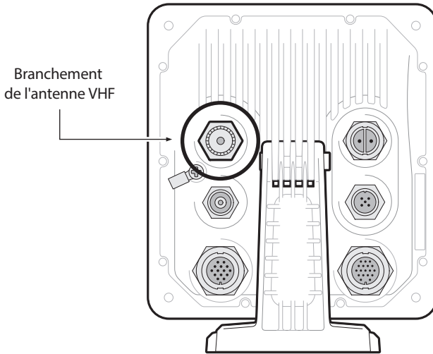
Figure 10 Branchement de l'antenne VHF
