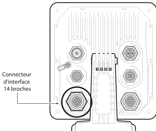
Figure 11 Connexion du port d'entrée de série
