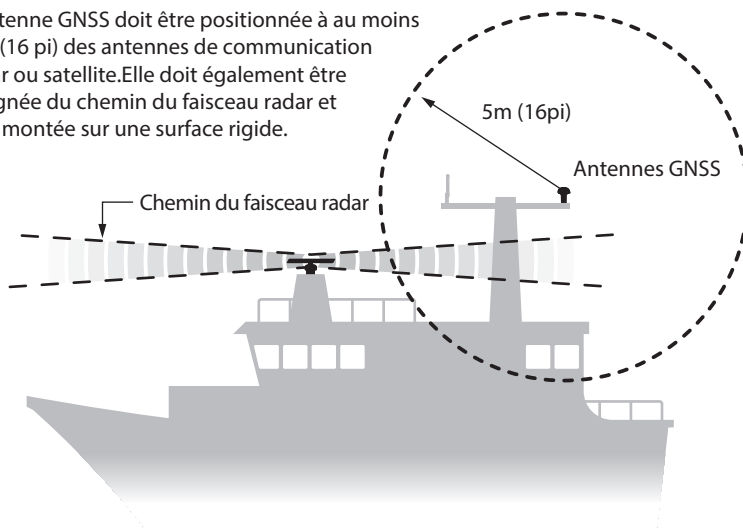
Figure 7 Emplacement de l'antenne GNSS
