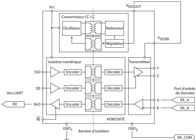
Figure 28 Schéma du port d'entrée
