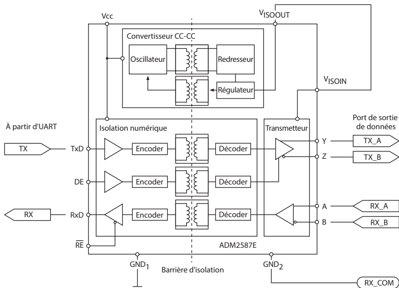
Figure 29 Schéma du port de sortie de données
