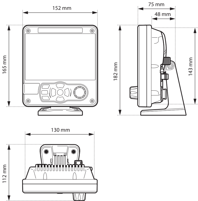
Figure 30 Dimensions de l'émetteur SIA
