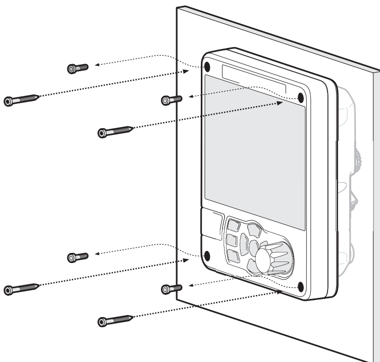
Figure 6 Installation sur panneau de l'émetteur SIA
