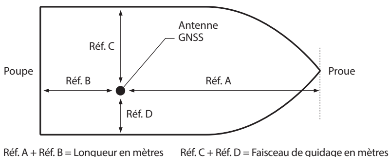
Figure 22 Mesure des dimensions du bateau
