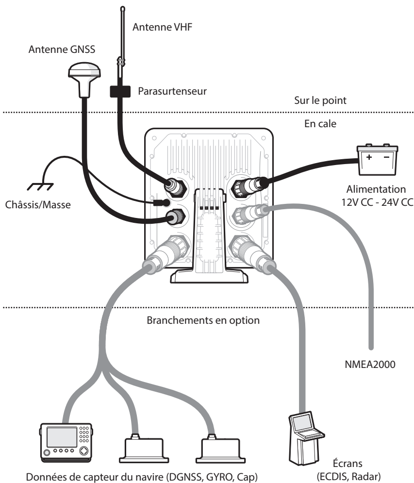
Figure 3 Connexion type de l'émetteur SIA
