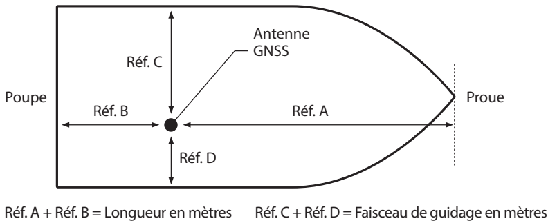
Figure 35 Position de l'antenne GNSS
