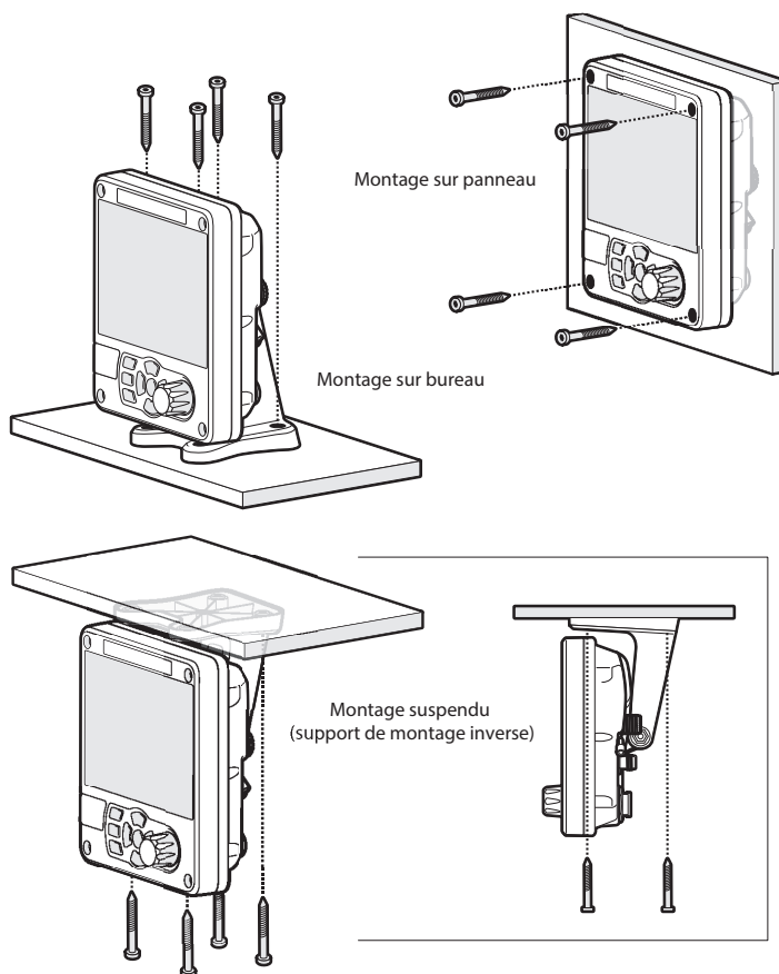
Figure 4 Installation de l'émetteur SIA
