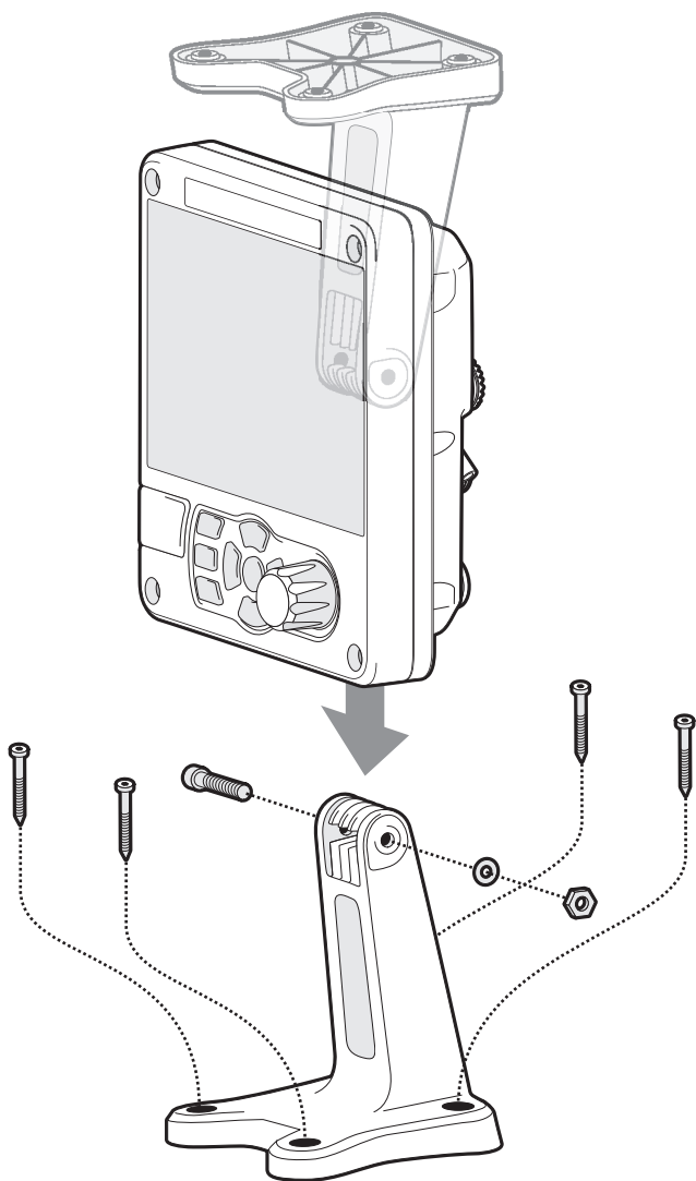
Figure 5 Installation sur bureau de l'émetteur SIA
