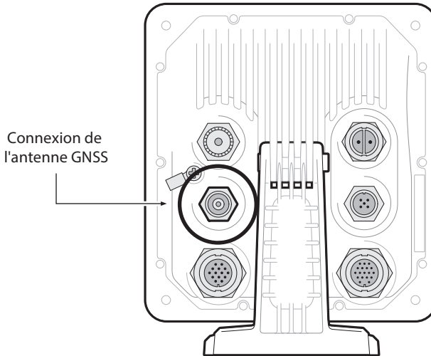
Figure 8 Connexion de l'antenne GNSS
