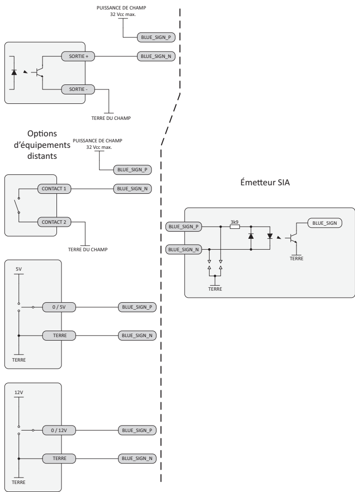
Figure 27 Options de raccordement de l'interface Signal bleu
