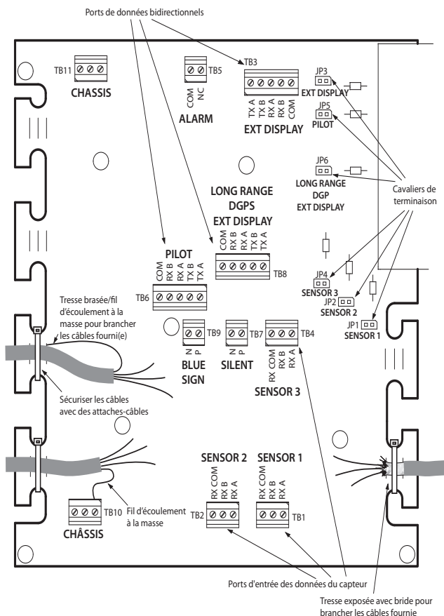
Figure 33 Raccordements de la boîte de connexion
