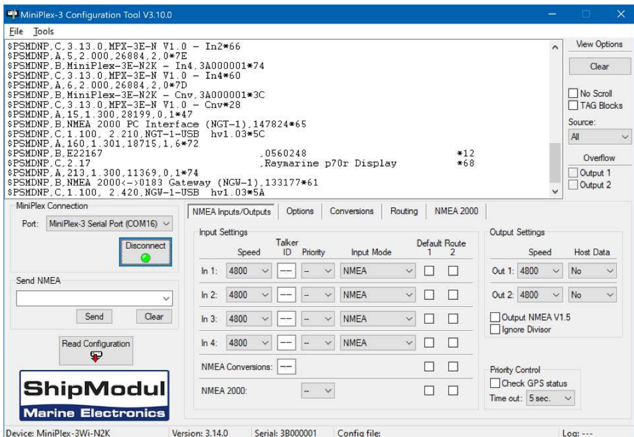
Figure 42: La fenêtre principale de l'utilitaire MPXConfig3
